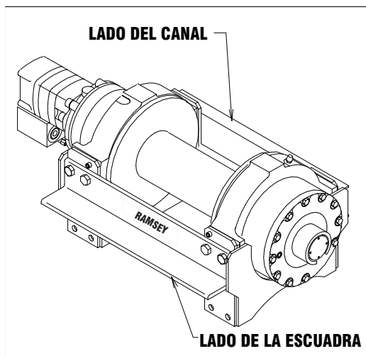
MONTAJE DERECHO
