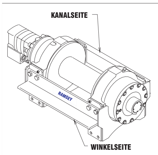
RECHTSSEITIGE MONTAGE
