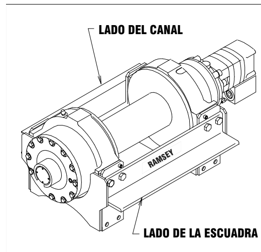
MONTAJE IZQUIERDO
