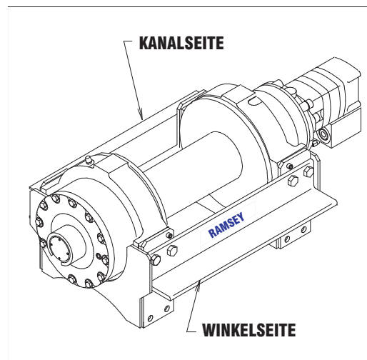
LINKSSEITIGE MONTAGE
