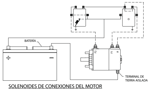
SOLENOIDES DE CONEXIONES DEL MOTOR
